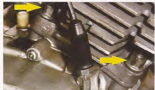
Tuercas que sujetan el cilindro al carter
